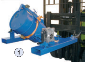
Pinza para bidones horizontal y vertical
