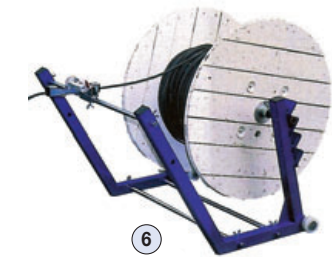
Opcional contador de cable, máximo Ø 22 mm. Ref. 12106
