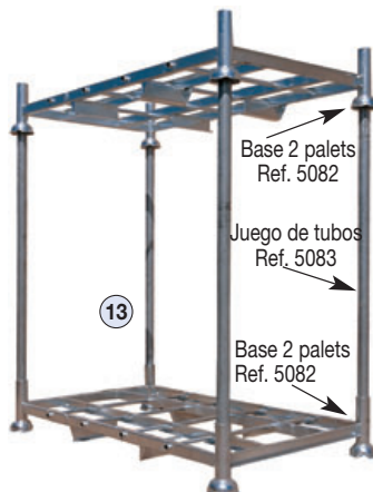
13 ESTANTERÍA DESMONTABLE PARA PALETS de hasta 1.000 x 1.200 Apilable hasta 4 alturas Carga 2.200 Kg
