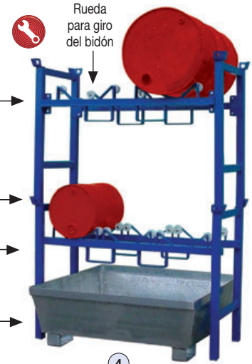
Rueda para giro del bidón Ref. 3035 Estanteria para 2 bidones de 200 litros Orejetas para apilar Ref. 3036 Estanteria para 3 bidones de 50 litros Ref. 3037-G Cubeta para ref. 3035 Ref. 3047-G Cubeta para Ref. 3036
