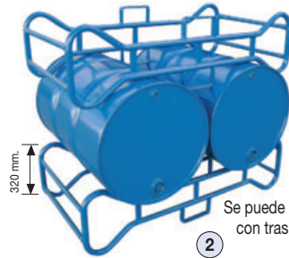
Rueda para giro del bidón Ref. 3035 Estanteria para 2 bidones de 200 litros Orejetas para apilar Ref. 3036 Estanteria para 3 bidones de 50 litros Ref. 3037-G Cubeta para ref. 3035 Ref. 3047-G Cubeta para Ref. 3036
